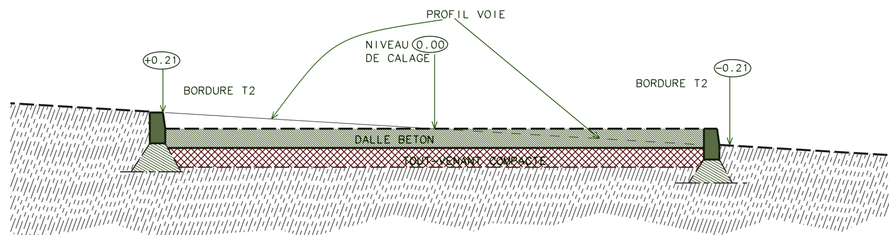
PROFIL CC
