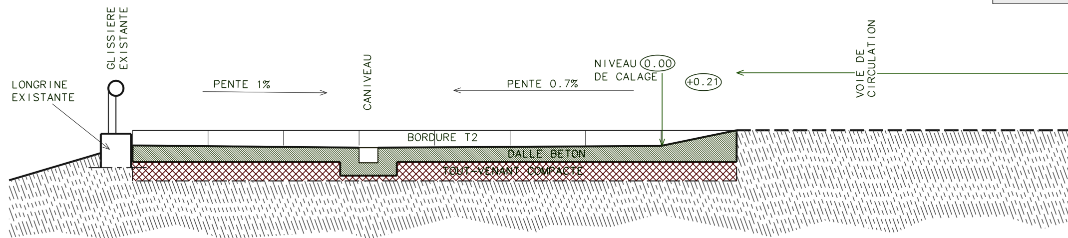
PROFIL AA
